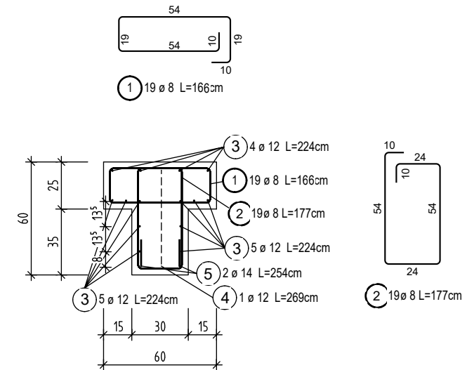
Seitenansicht
