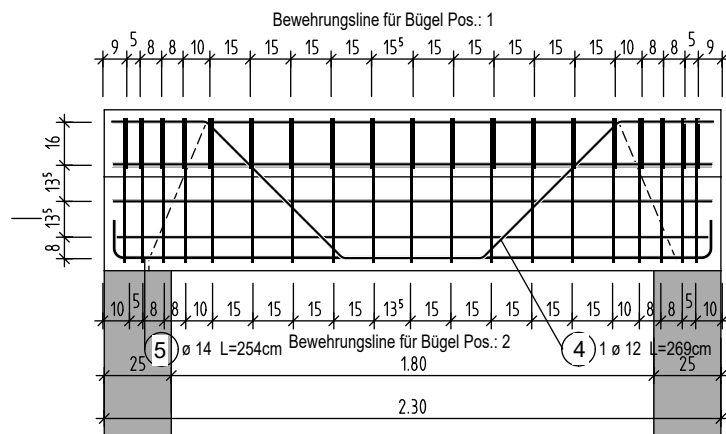
Vorderansicht
